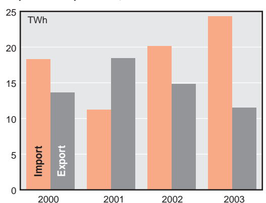
Import och export av el, TWh
