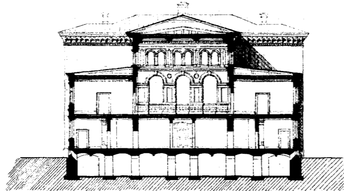
Section A-B
