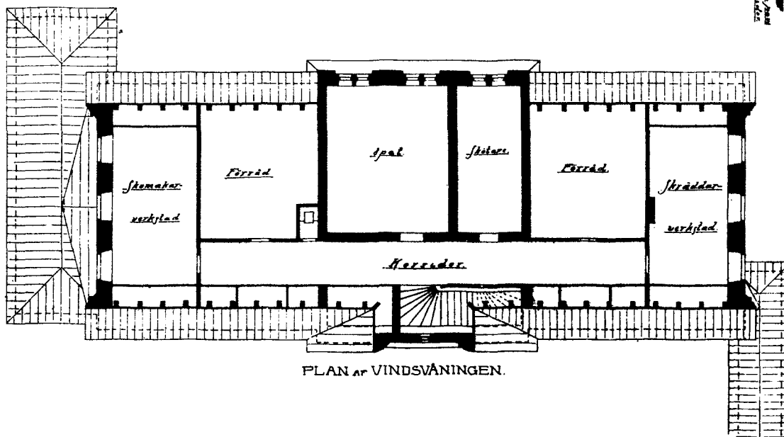
PLAN av VÅNINGEN 1 TR. UPP.
