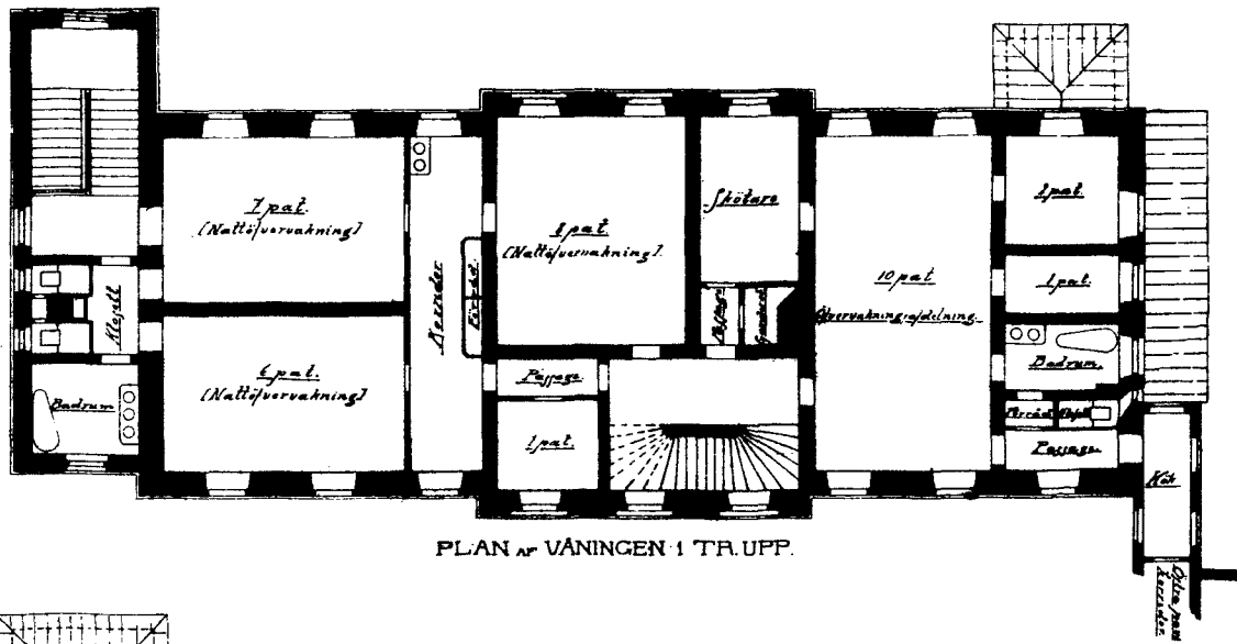
PLAN av BOTTENVÅNINGEN.
