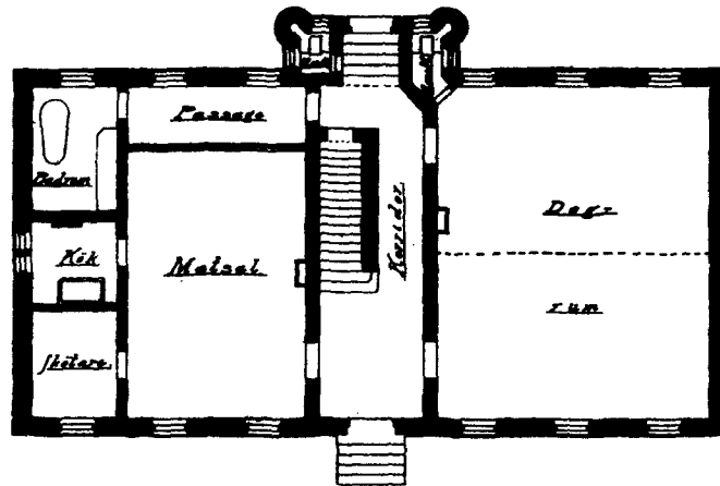
PLAN AF BOTTENVÅNINGEN.
