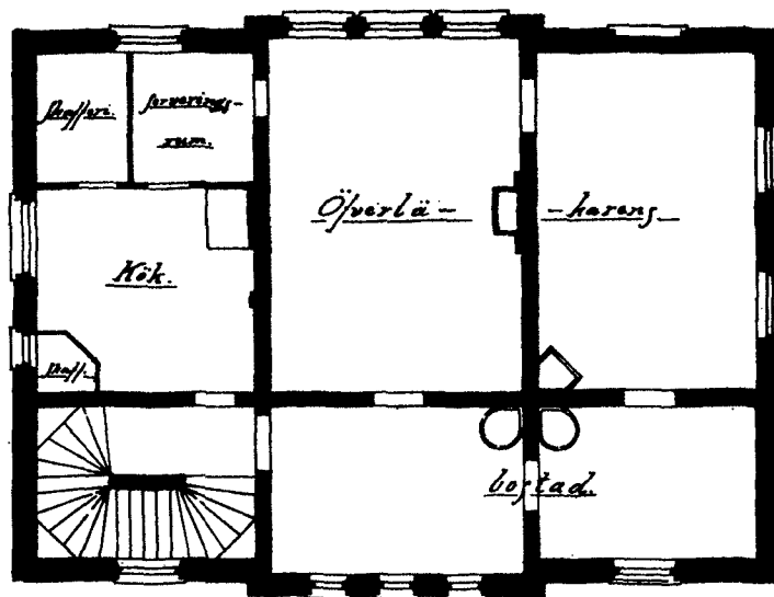
PLAN AF VÅNINGEN 1 TR. UPP.
