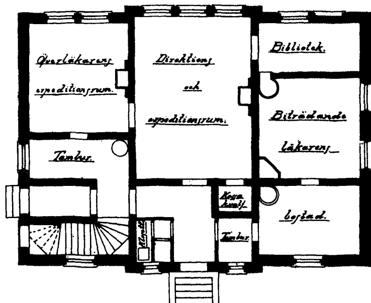
PLAN AF BOTTENVÅNINGEN.
