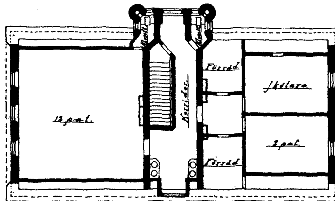
PLAN AF VINDSVÅNINGEN.
