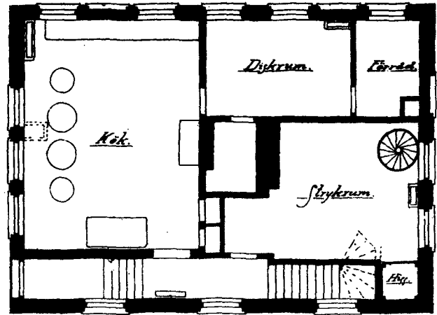
PLAN AF VÅNINGEN 1 TR. UPP.
