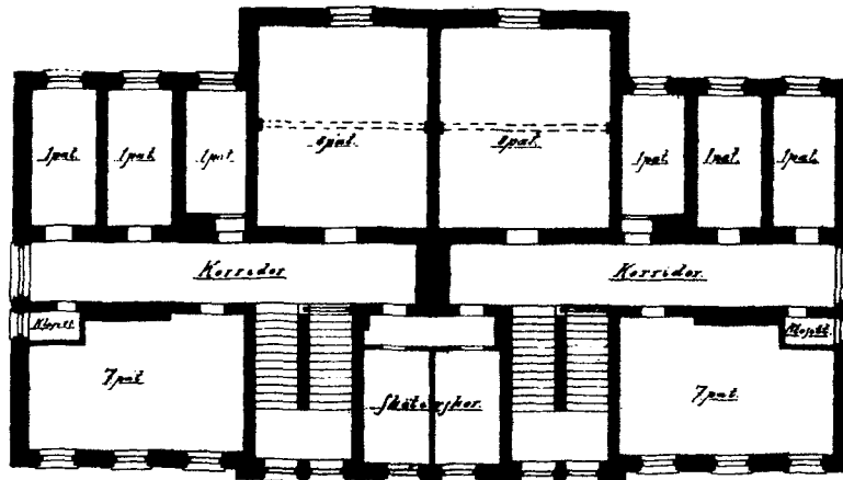
PLAN af VÅNINGEN I TR. UPP.
