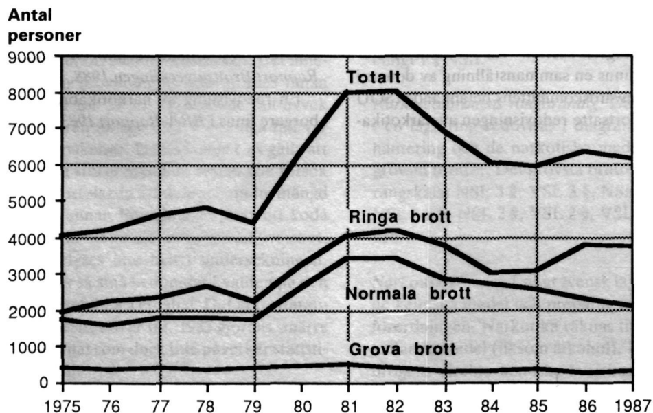
Diagram 3.7.2 För narkotikabrott lagförda personer, 1975–1987, efter brottsrubricering Persons found guilty of drug offences, 1975–1987, by seriousness of the offence
