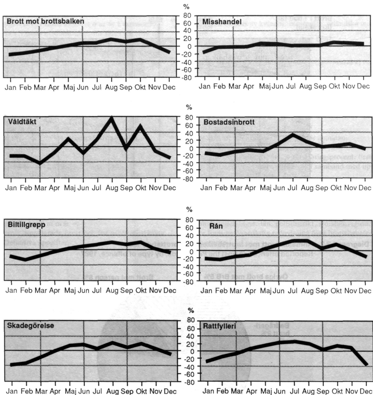
Diagram 3.2.3 Procentuella variationer i antalet anmälda brott för vissa brottstyper, 1987
