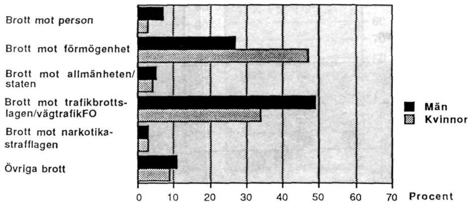
Diagram 3.4.4 Personer som lagförts, efter huvudbrott, 1987. Brottsgrupperna fördelade efter kön, ålder och medborgarskap. Procentuell fördelning Persons found guilty, by principal crime, 1987. Crime categories distributed by sex, age and citizenship, in percent
