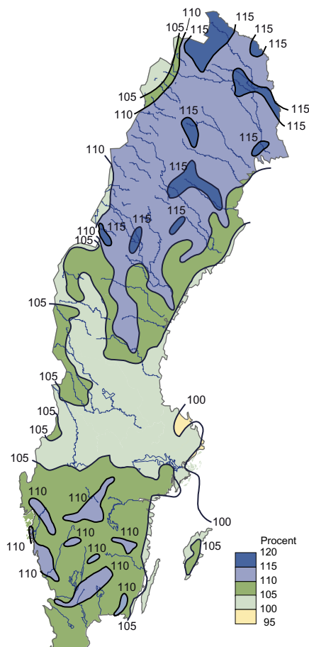
Nederbördsförändringar från perioden 1961–1990 till 1991–2005
