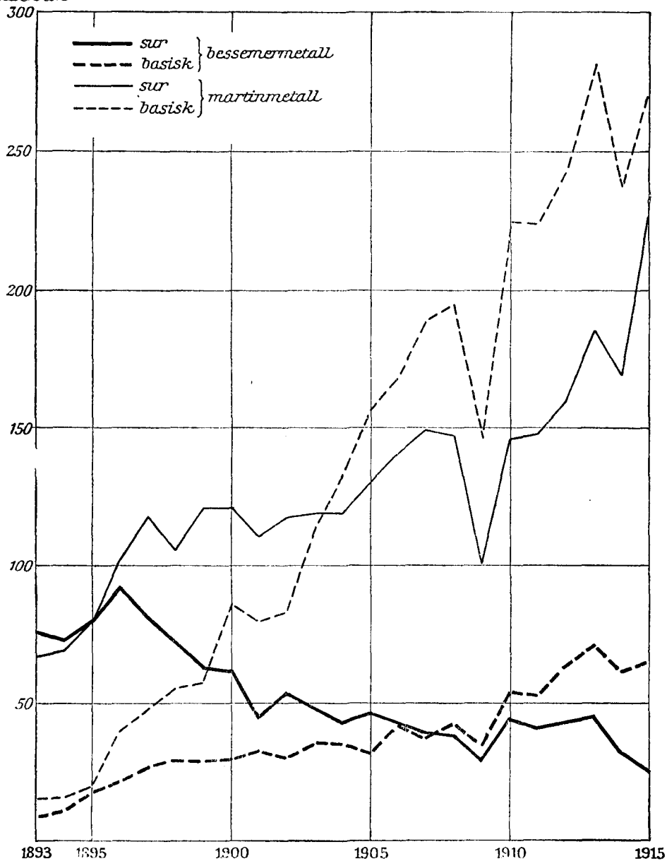
Diagram 26. Tillverkning av götejärn av olika slag, åren 1893—1915.
