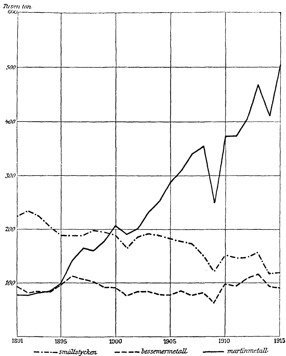
Diagram 25. Tillverkning av smidbart järn och stål, åren 1891—1915.
