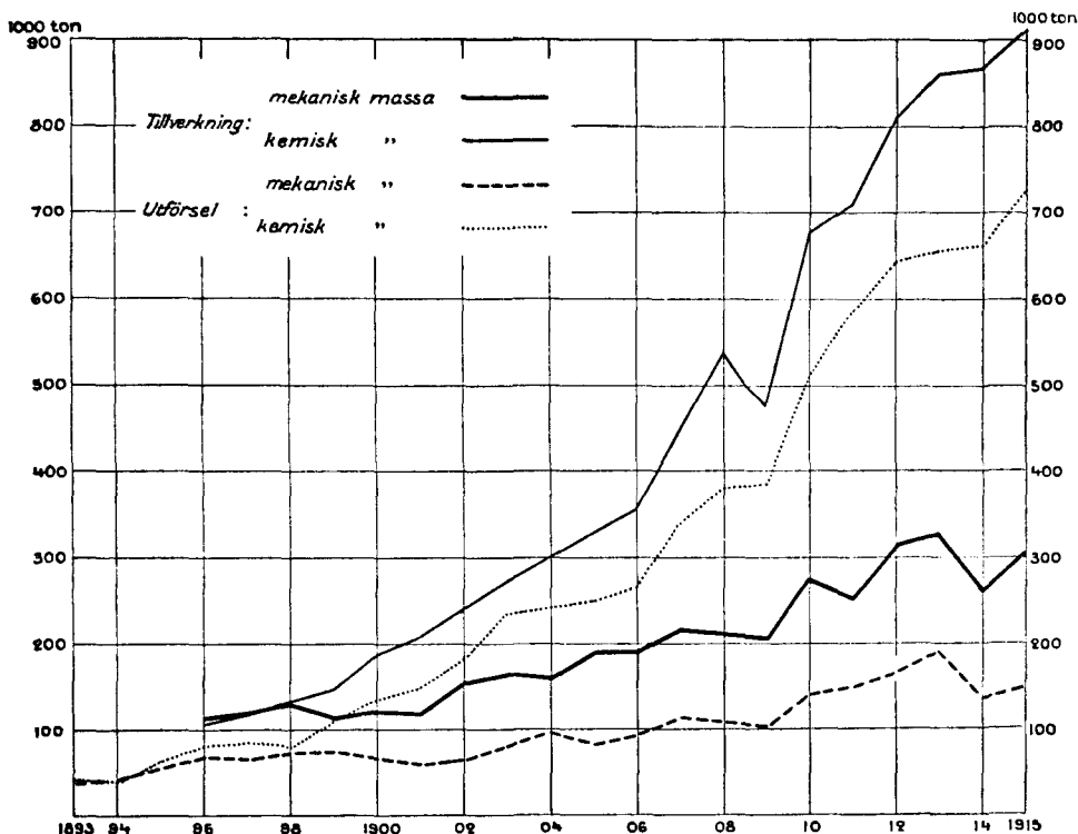
Diagram 18. Tillverkning och utförsel av pappersmassa, åren 1893–1915.
