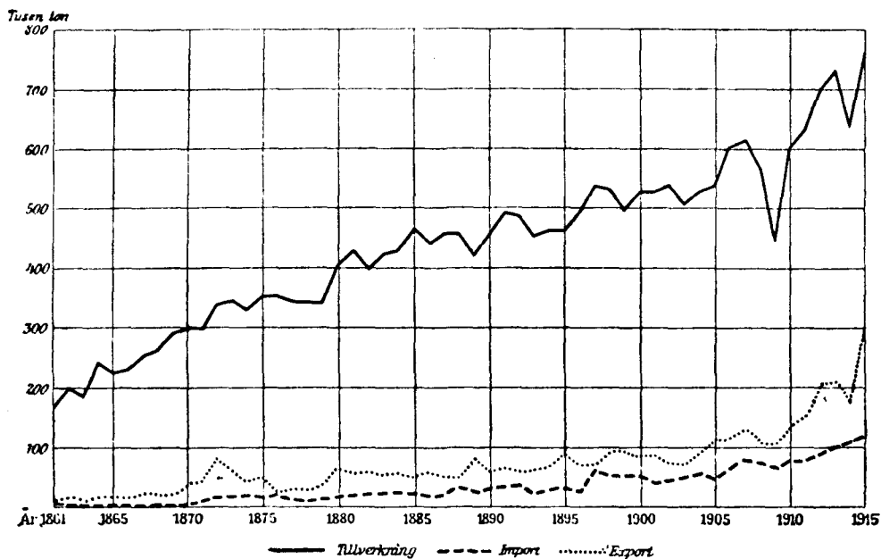
Diagram 24. Tillverkning, import och export av tackjärn, åren 1861–1915.
