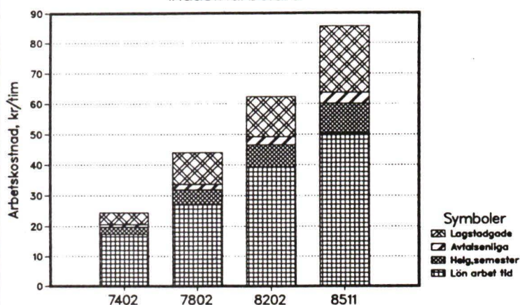
Arbetskraftskostnader 1974-1985 Industriarbetare
