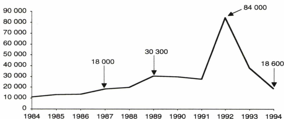
Figur 3 Antalet asylsökande 1984–1994
