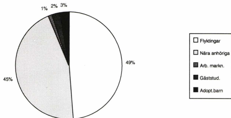
Figur 2 Invandringens sammansättning 1980–1994
