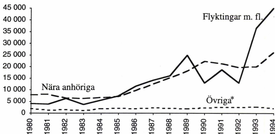
Figur 1 Beviljade uppehållstillstånd 1980–1994
