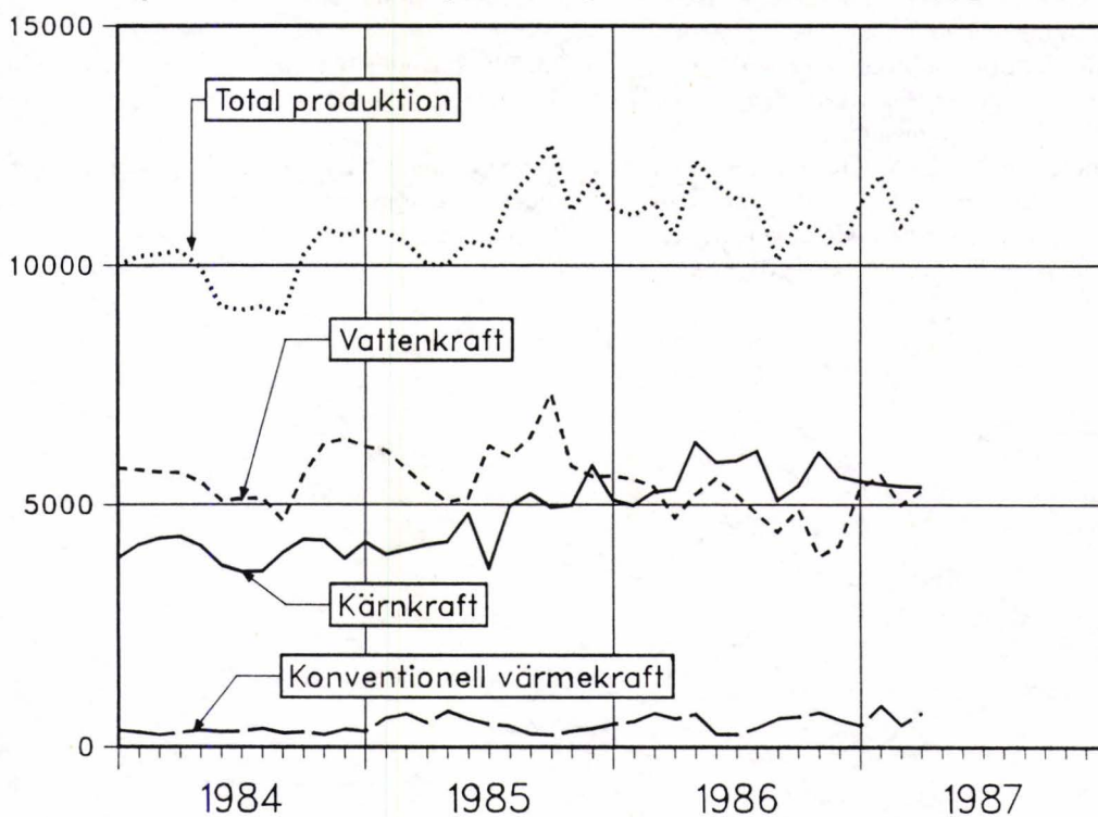
Elproduktionen fördelad på kraftslag. Säsongsrensade månadsuppgifter. GWh
