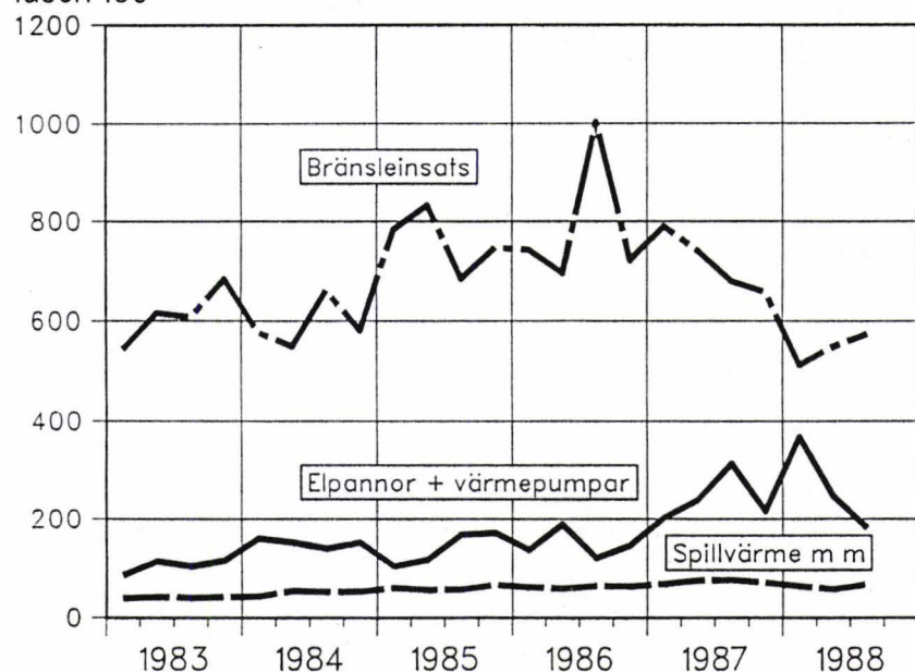
Energiinsats för fjärrvärmeproduktion 1a kv 1983–3e kv 1988, säsongrensade värden
