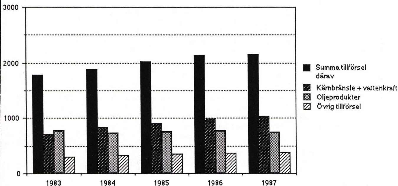
Bruttotillförsel av energi, PJ
