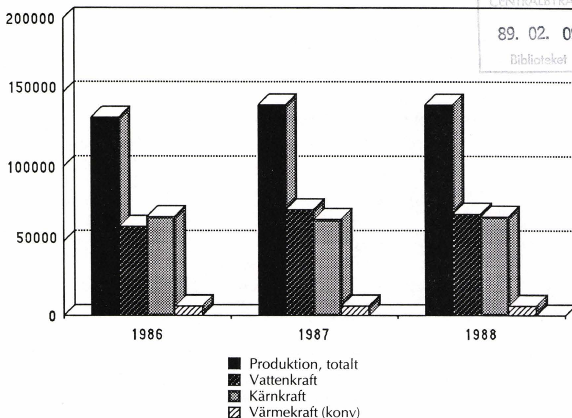
Elproduktion fördelad på kraftslag, GWh
