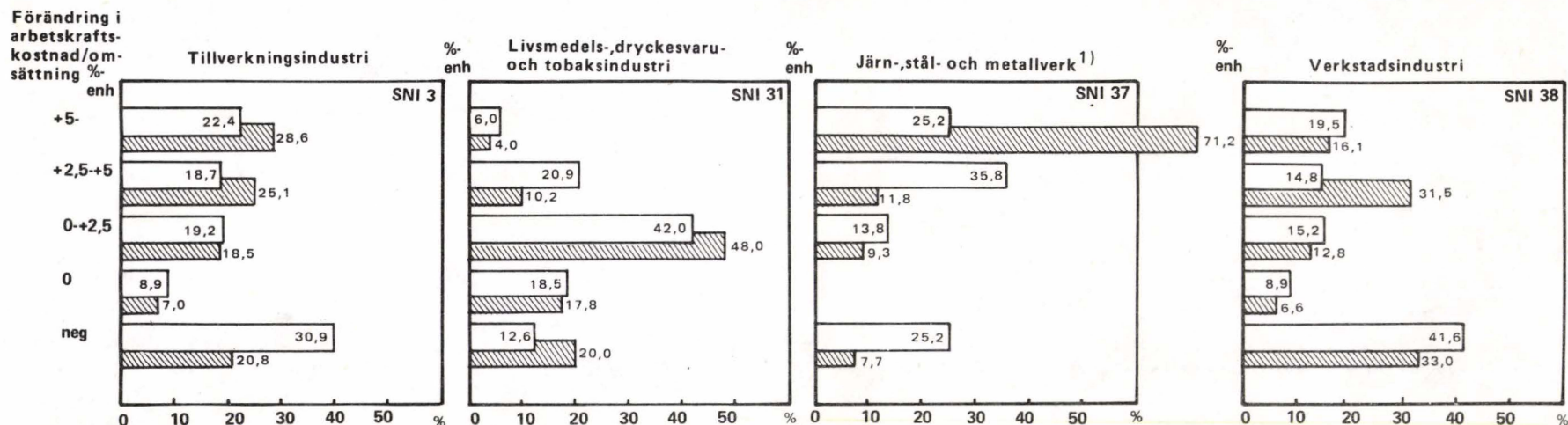
Diagram 4:3 Industriföretagen grupperade efter förändring i arbetskraftskostnad i procent av omsättning mellan 1974 och 1975
