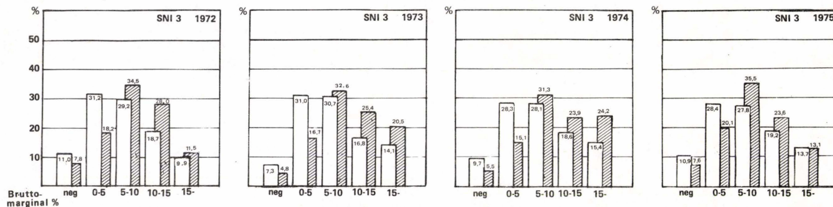
Diagram 1:1 Industriföretagen grupperade efter bruttomarginal 1972 - 1975
