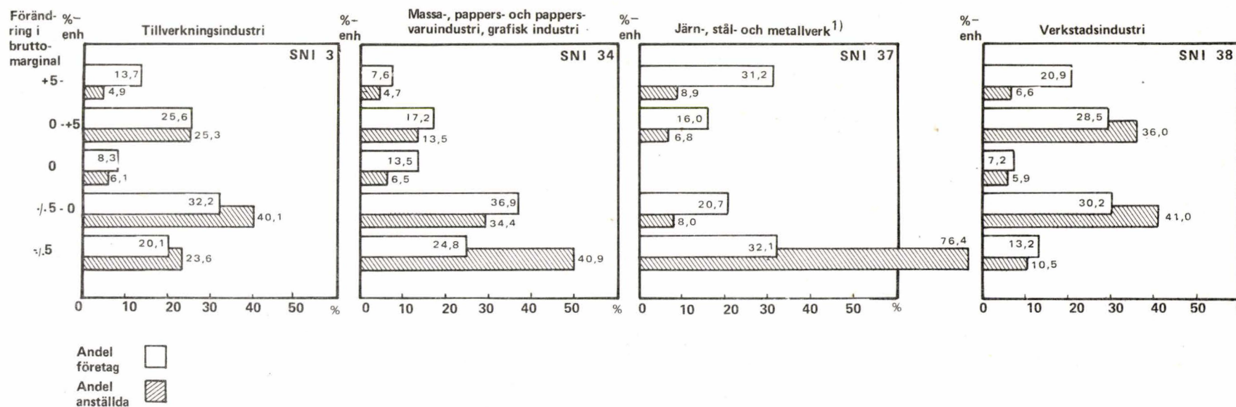
Diagram 4:2 Industriföretagen grupperade efter förändring i bruttomarginal mellan 1974 och 1975
