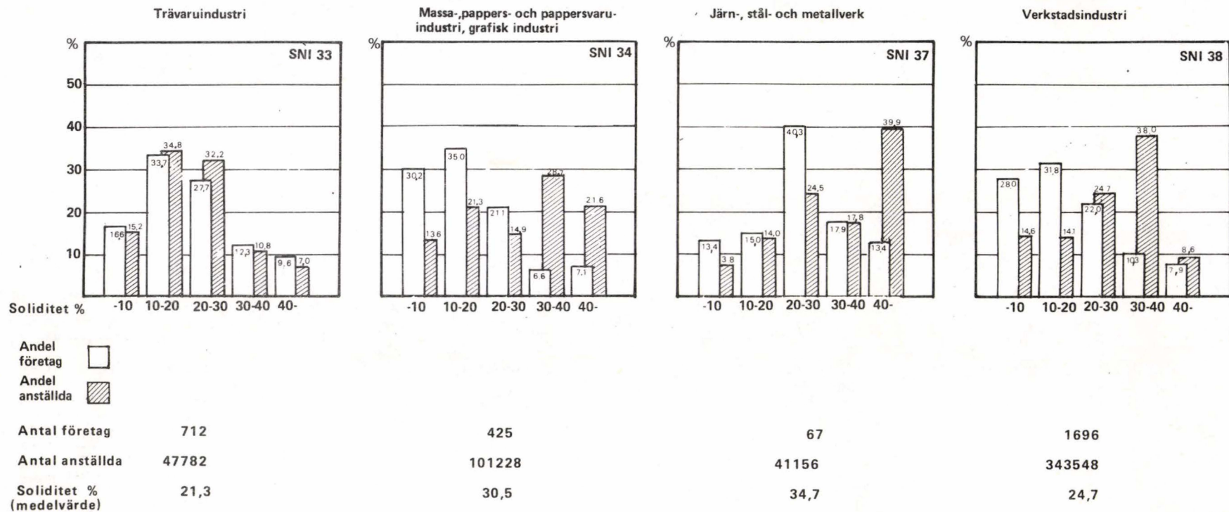
Diagram 2:3 Industriföretagen grupperade efter soliditet 1975
