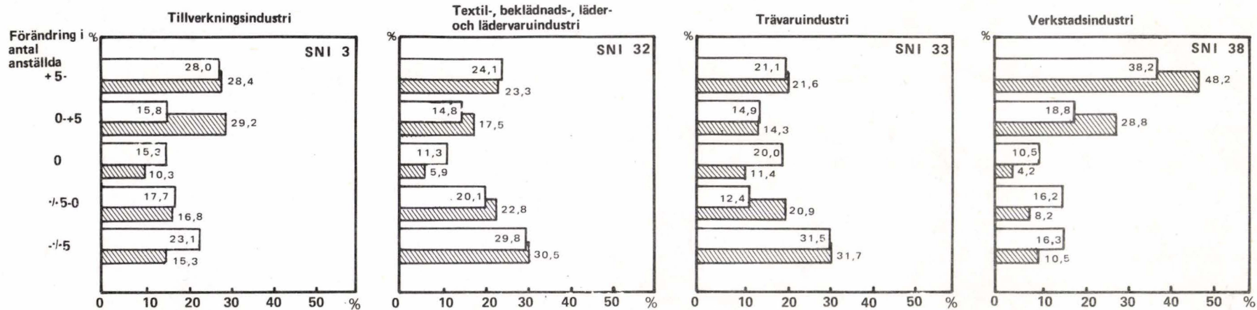
Diagram 4:1 Industriföretagen grupperade efter förändring i antal anställda mellan 1974 och 1975
