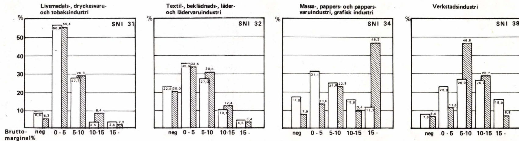
Diagram 2:1 Industriföretagen grupperade efter bruttomarginal 1975
