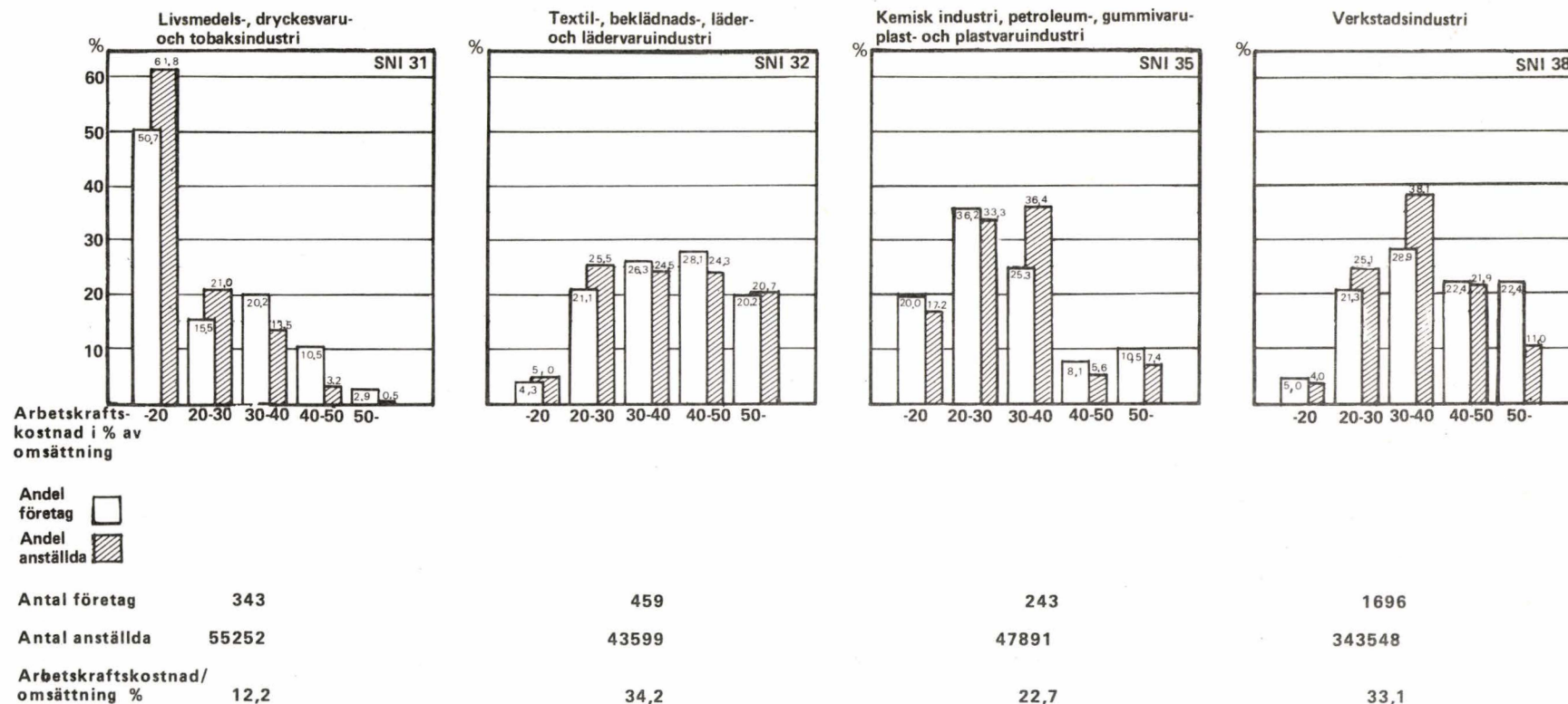
Diagram 2:2 Industriföretagen grupperade efter arbetskraftskostnad i procent av omsättning 1975
