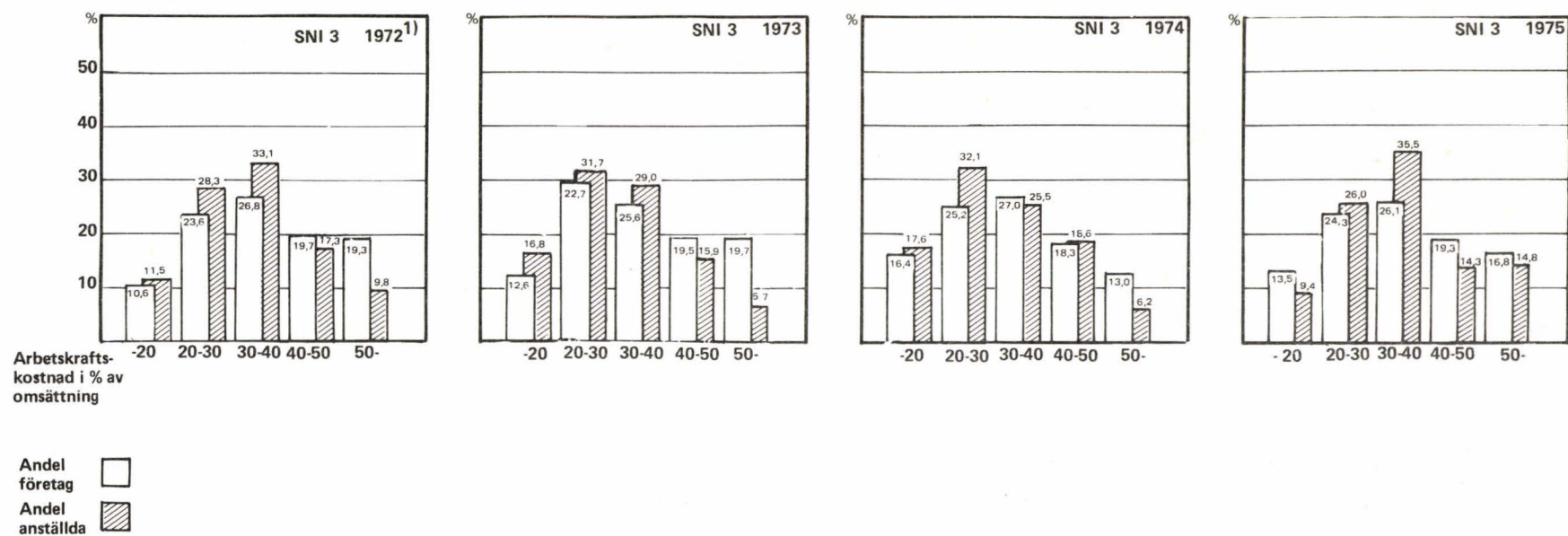
Diagram 1:2 Industriföretagen grupperade efter arbetskraftskostnad i procent av omsättning 1972 – 1975
