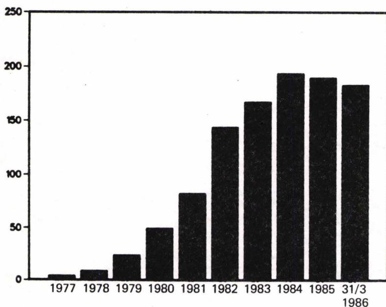
Sveriges nettoskuld till utlandet per 31 december åren 1977 till 1985 samt 31 mars 1986. Miljarder kronor.
