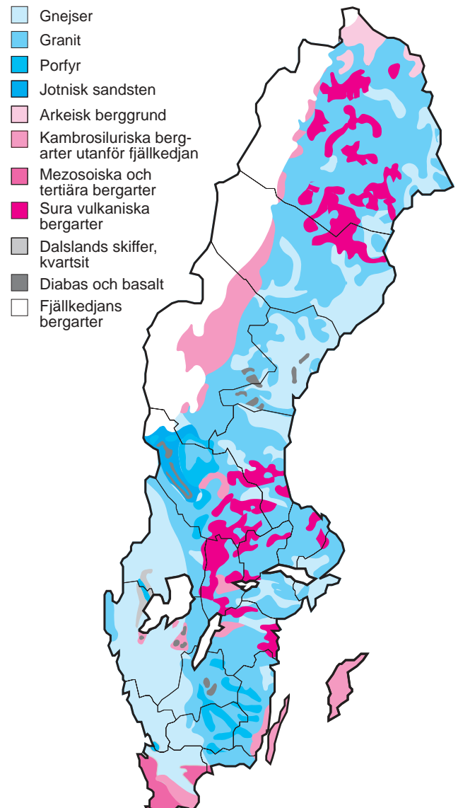
Figur 10 Berggrund
