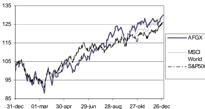
Affärsvärldens generalindex, MSCI World och Standard&Poor 500 under 2003, indexerat 2002-12-30=100
